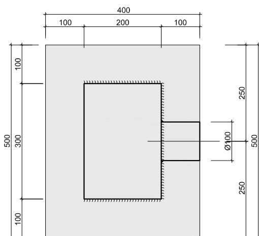
WIDOK OD TYŁU
