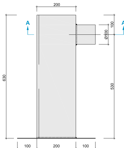
WIDOK BOCZNY
