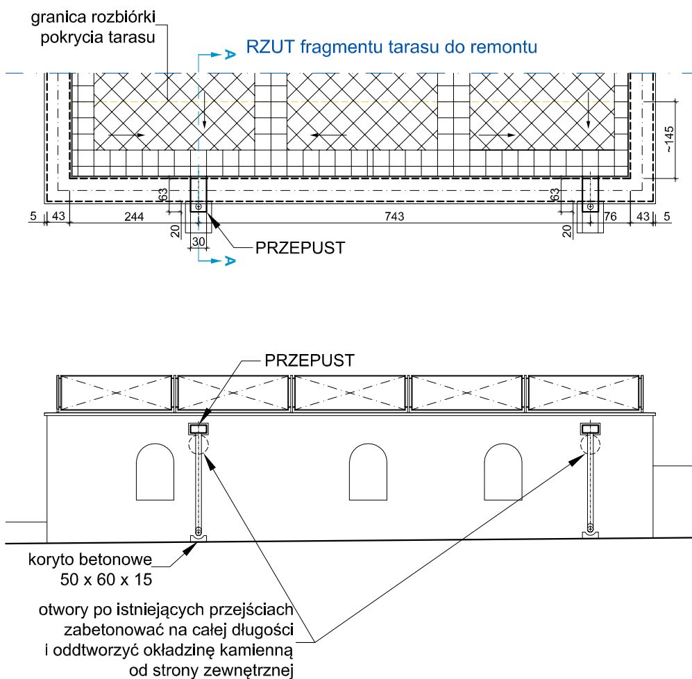
ELEWACJA FRONTOWA TARASU
