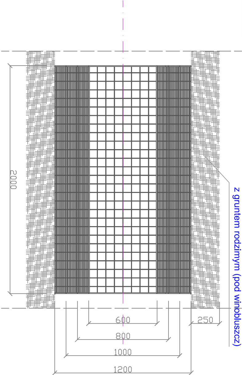
Rzut kosza
