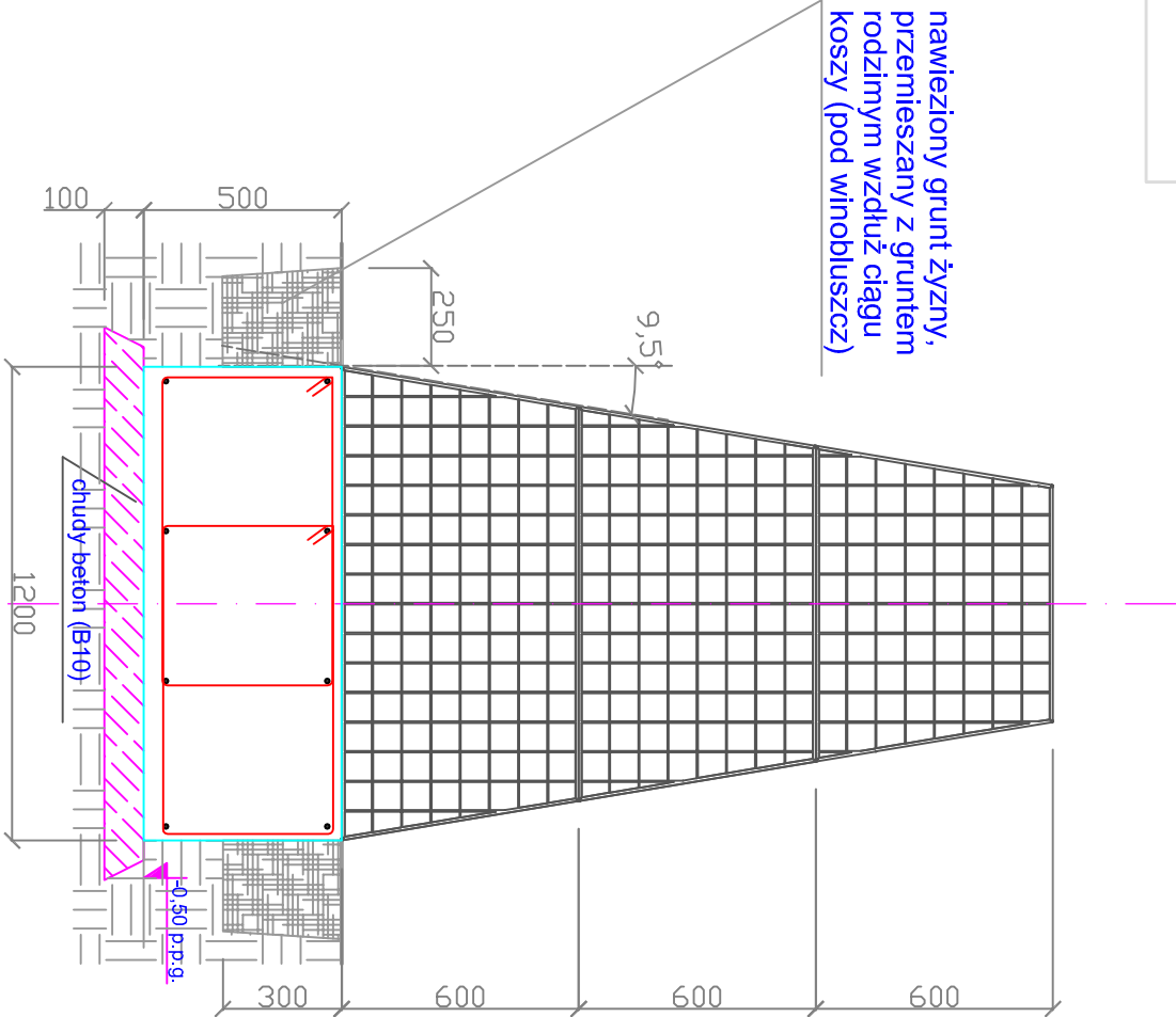
Profil kosza
