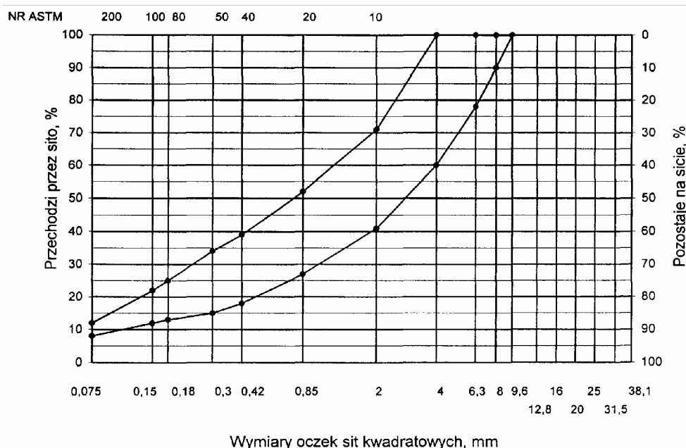
Rys. . Krzywe graniczne uziarnienia mieszanki mineralnej BA od 0 do 8mm, od 0 do 6,3 mm do warstwy ścieralnej nawierzchni drogi o obciążeniu ruchem nawierzchni drogi o obciążeniu ruchem KR1 lub KR2
